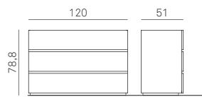
Elemento 3 cassetto P=51 H=78,8
