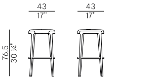
942/AC sgabello \ stool
